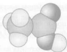
Рис. 10.7. Модель молекулы уксусной кислоты
