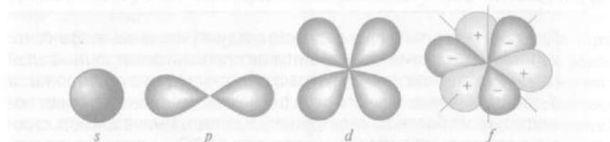
Рис. 2.2. Форма s -, p -, d - и f -электронных облаков
